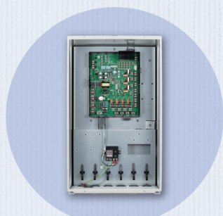
マルチコントローラ FMC-03 内部
